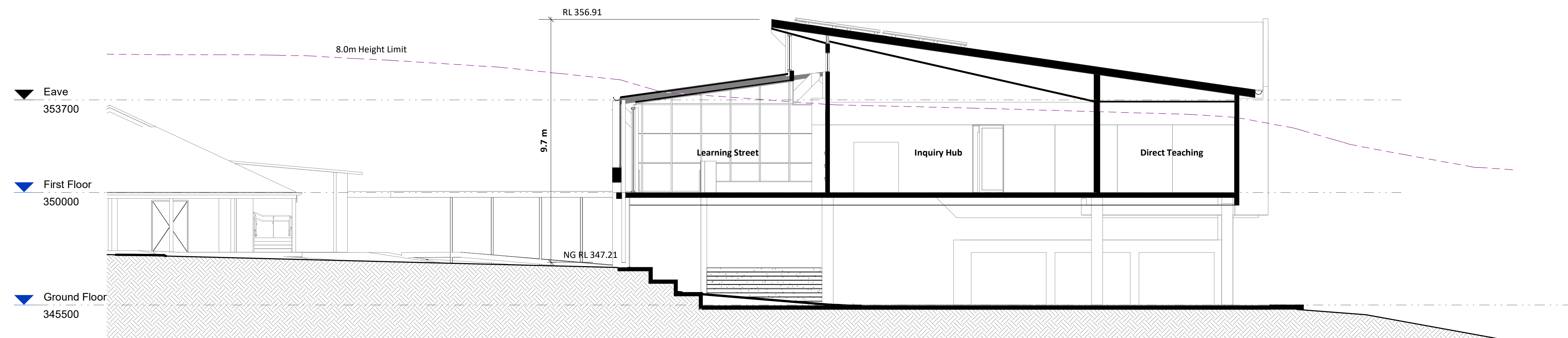
3 Cross Section 3 1 : 100
