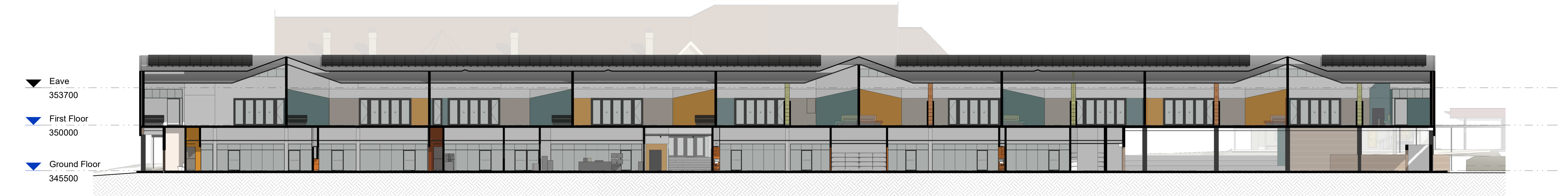
3 Long Section C 1 : 200
