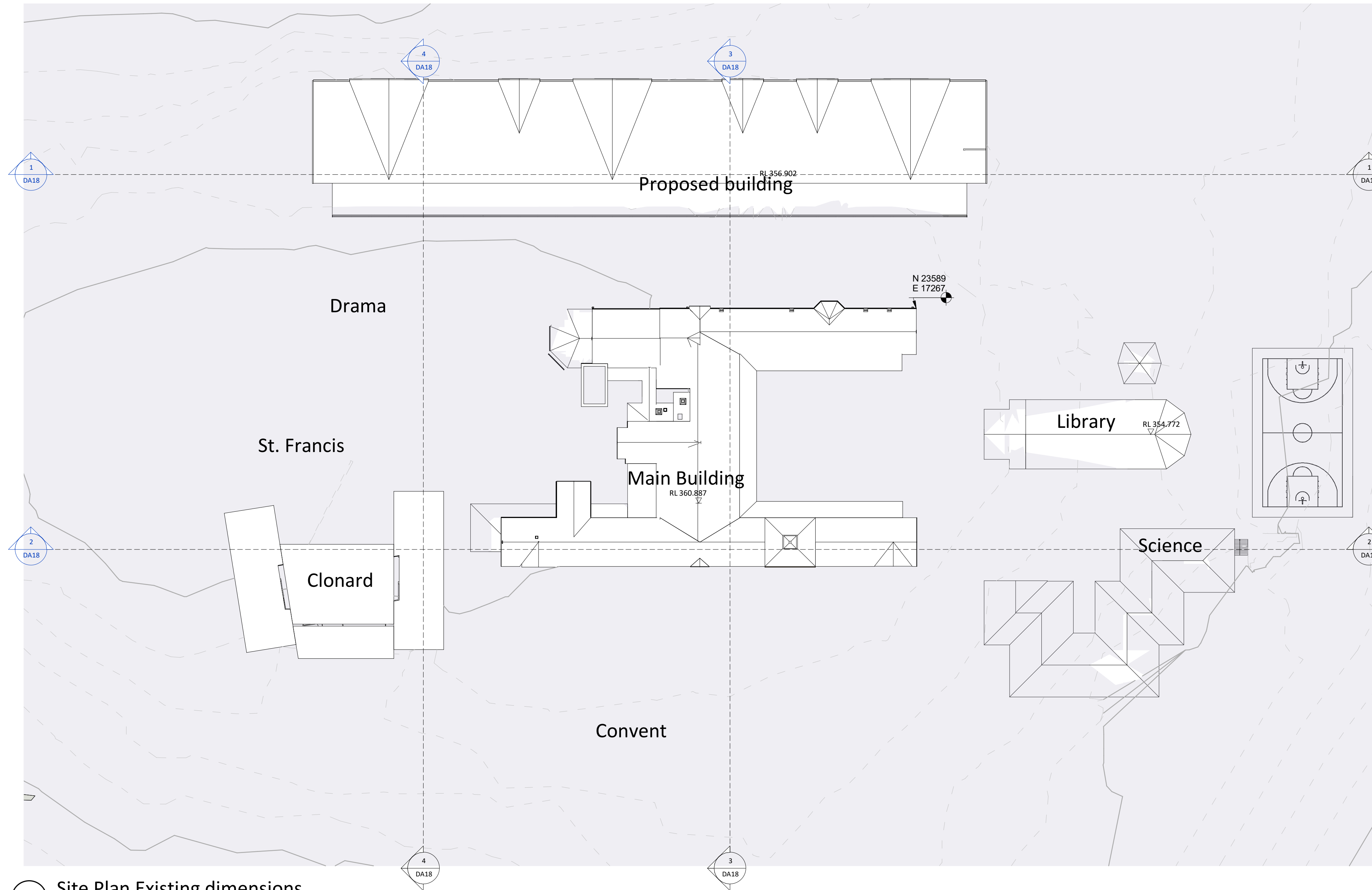
01 Site Plan Existing dimensions 1 : 500
