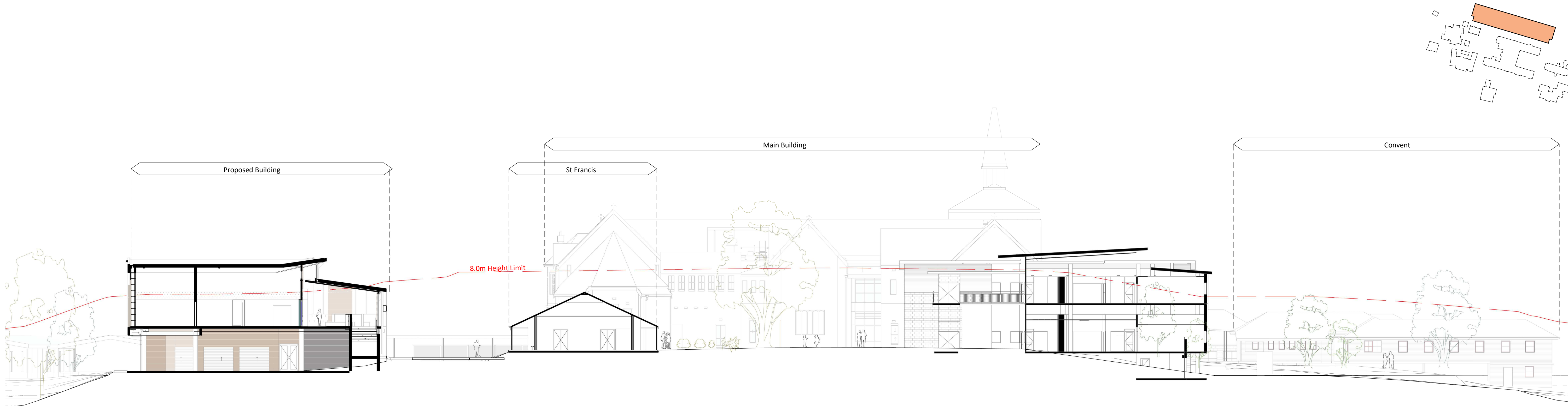
1 Site Section 1 1 : 200
