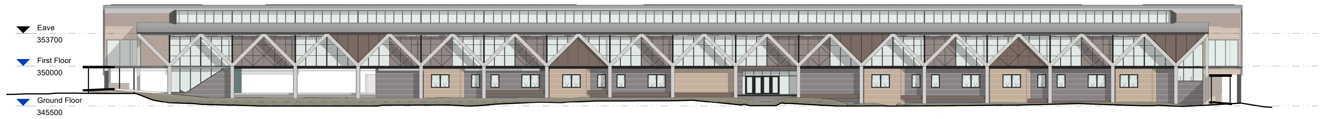
2 Elevation - South DA 1 : 200
