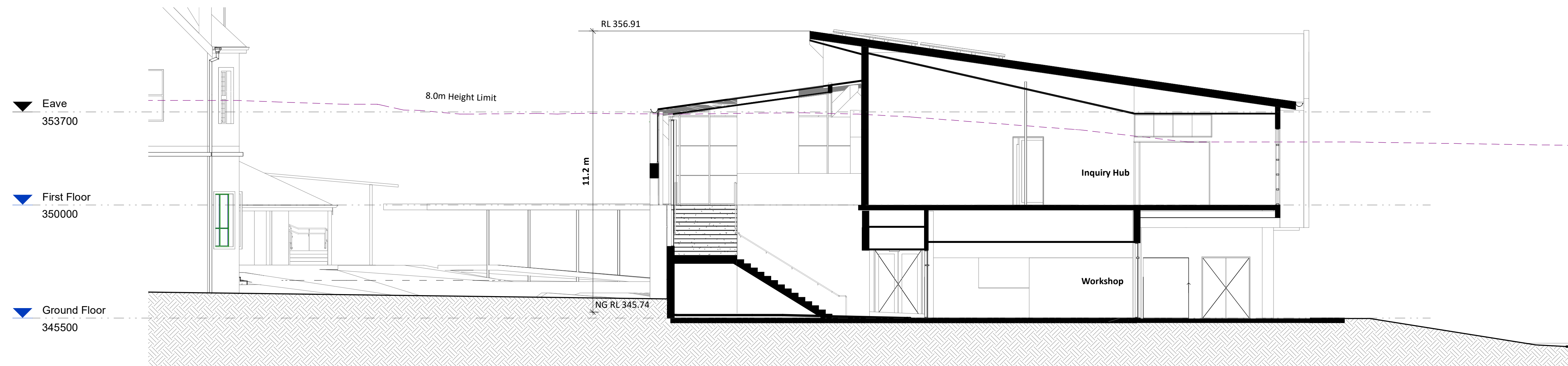
1 Cross Section 1 1 : 100
